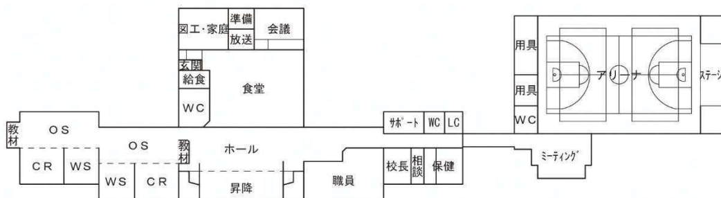
1 階 平 面
