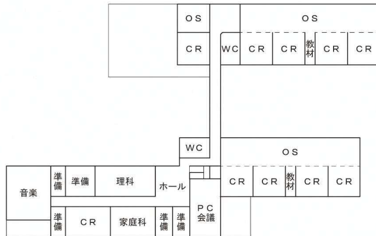
2 階 平 面
