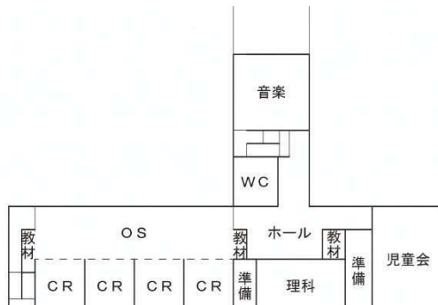
3 階平面
