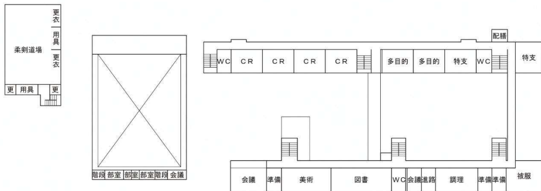
2 階 平 面
