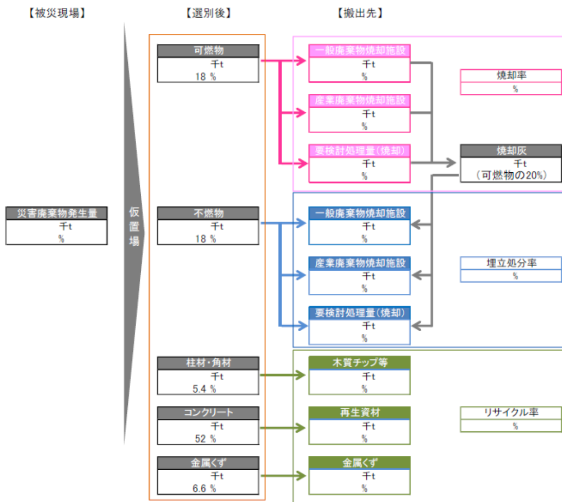
図 1 1 災害廃棄物の基本処理フロー
