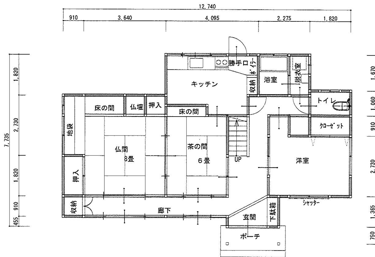
1 階平面図 1/100
